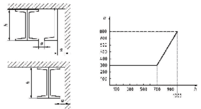
Bild C.1 – Mindestabstände bei engen Abständen zwischen Oberflächen gemäss Norm SN EN ISO 12944-3:2017
