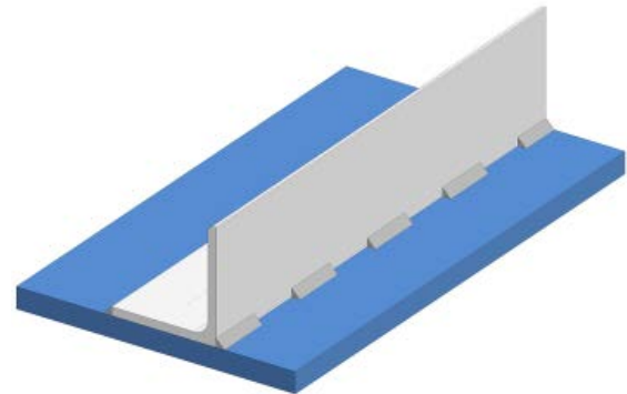
Abb. 14.1: Ungünstige Lösung, da nicht durchgeschweisst
