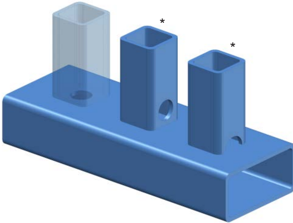
Abb. 11.1: * Die sichtbaren Entlüftungslöcher sind ungünstig, da Zinkschnäuze entstehen können
