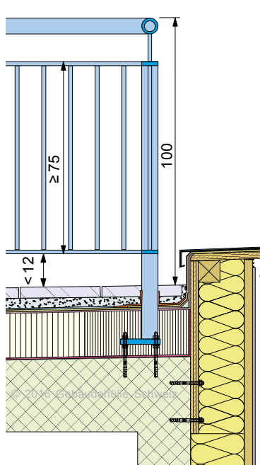
Abb. 10: Höhe von Schutzelementen und Öffnungen in Schutzelementen. Druckfeste Dämmung im Bereich der Konsole ca. 40 x 40 cm als druckfester Untergrund für die Flüssigkunststoffabdichtung empfehlenswert
