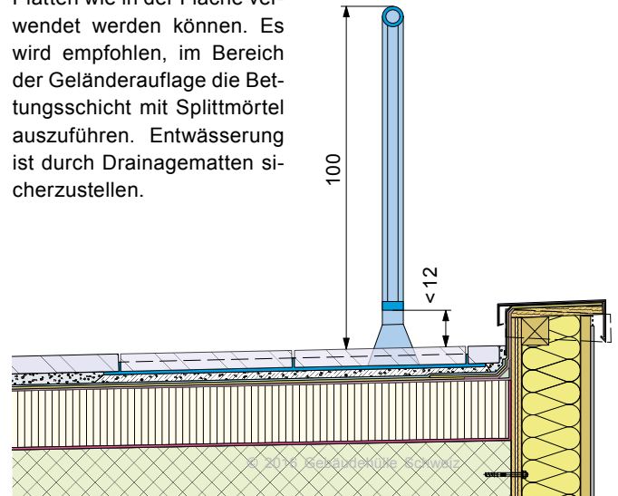
Abb. 19: Systemgeländer mit Auflast der Nuttschicht. Systemanforderungen beachten
